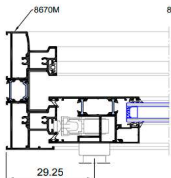
Sección A-A'
