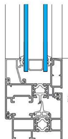
Sección Vertical
