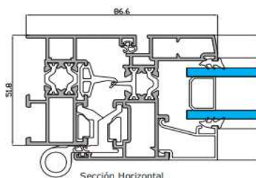
Sección Horizontal
