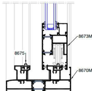
Sección B-B'
