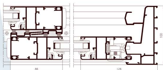
Sección
