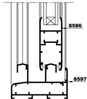
Sección B-B
