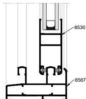
Sección B-B'
