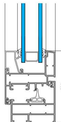
Sección Vertical
