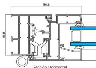
Sección Horizontal
