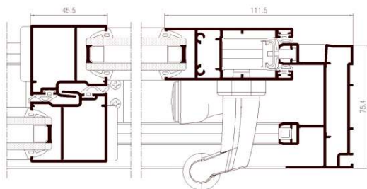
SIN ROTURA
