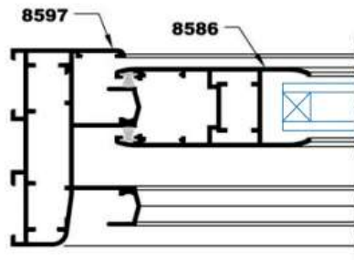
Sección A-A
