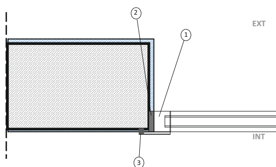
1: Cerco 2: Elastiflex 3: Iso Bloco 600
