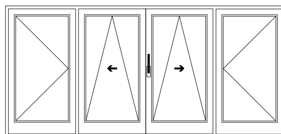
Esquema C – con travesaños centrales
