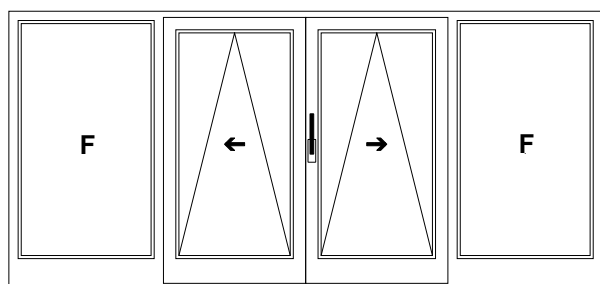
Esquema C – con travesaños centrales
