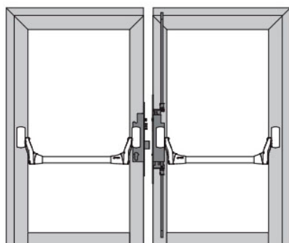
Antipánico 2 hojas con 1 y 2 puntos de cierre Cierre lateral 1 punto + superior e inferior
