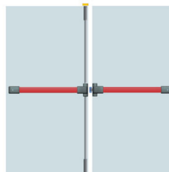
Antipánico 2 hojas con 1 y 2 puntos de cierre Cierre lateral + Cierre superior e inferior
