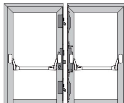
Antipánico 2 hojas con 3 y 2 puntos de cierre Cierre lateral 3 puntos + superior e inferior
