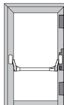
Antipánico 1 hoja con 3 puntos de cierre Cierre lateral 3 puntos
